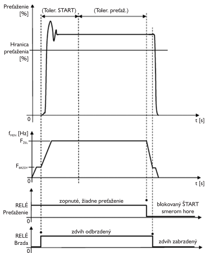
Obr.2 Preťažovací vypínač
