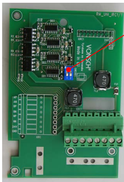
Rozšiřovací modul RM-UNI_IRC1 pre pripojenie s frekvenčným meničom UNIFREM 400
