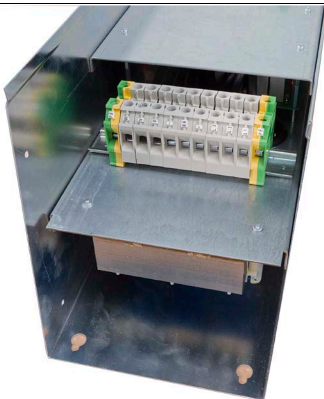
Pohľad na pevnú silovú svorkovnicu X0
